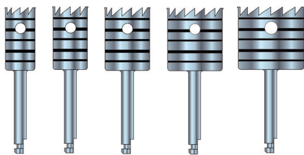
深度ライン：2-4-6-8-10mm
