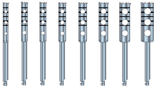
深度ライン：2-4-6-8-10mm
