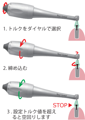
トルク選択ダイヤル (トルク値：7種10/15/20/25/30/32/35N-cm)
